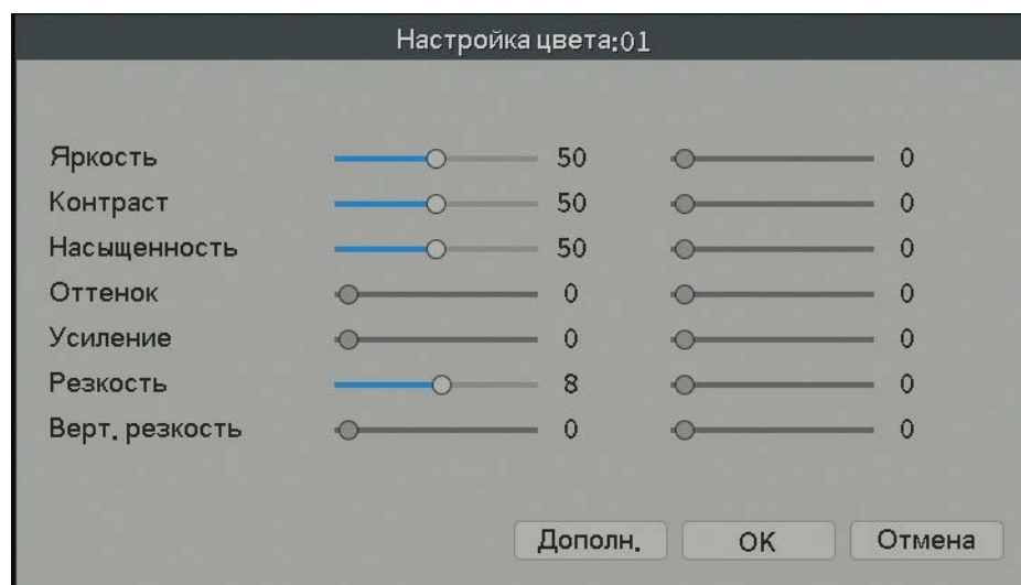
Рис.3.13 Настройки цвета
